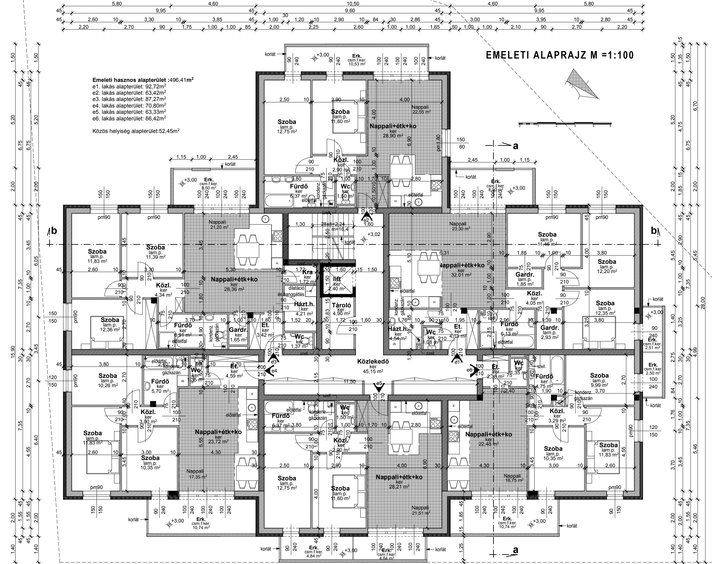
5 - 2 emeleti alaprajz m=1:100
